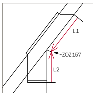
Toit avec jambette
